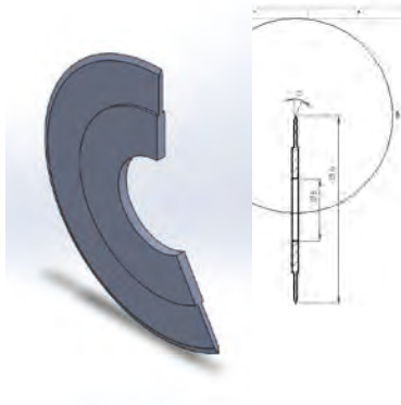
Quetschmesser
