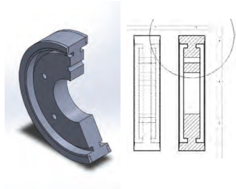
Doppelnutmesser
