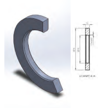
Zwischenringe
